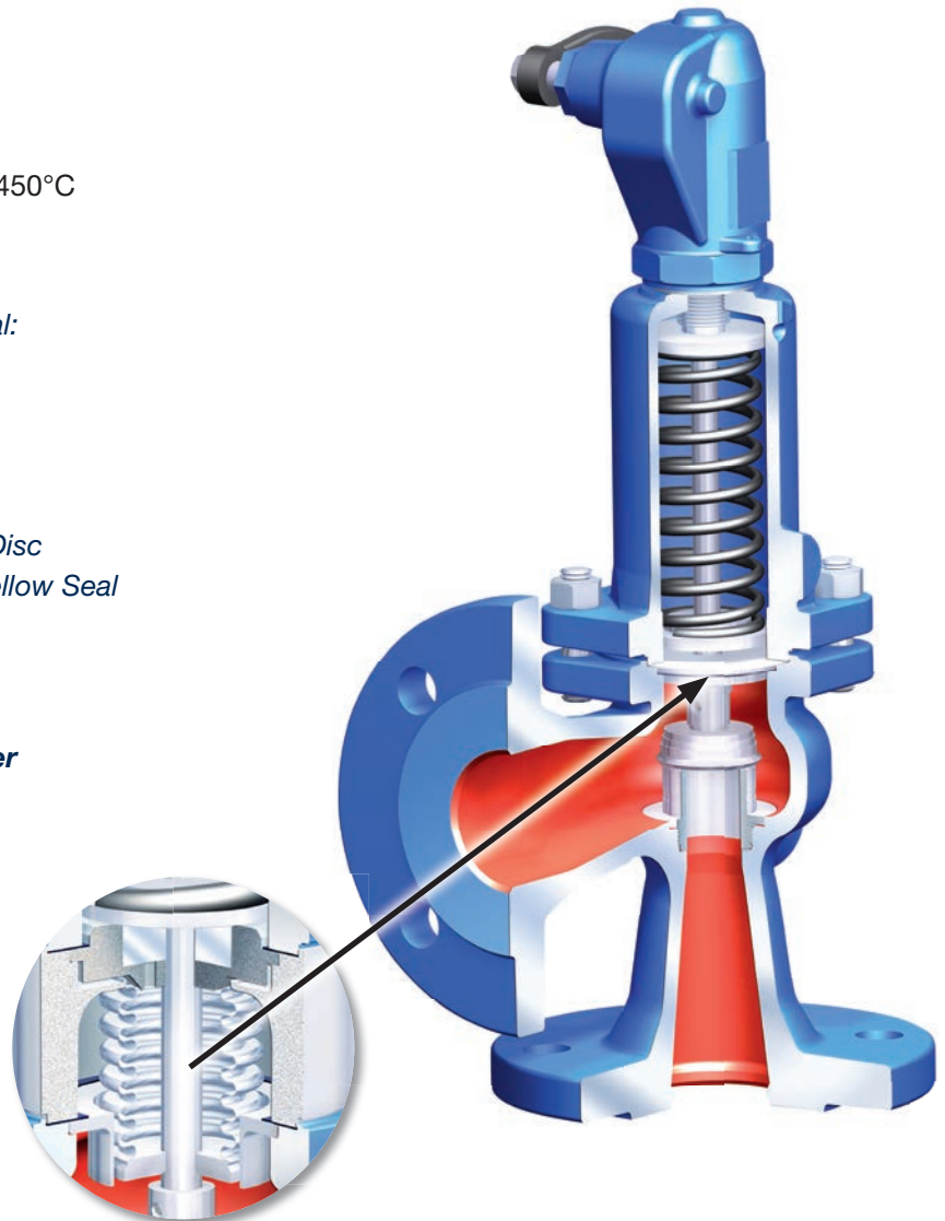
Optionaler Edelstahl Faltenbalg / Optional Stainless Steel Bellow Seal
