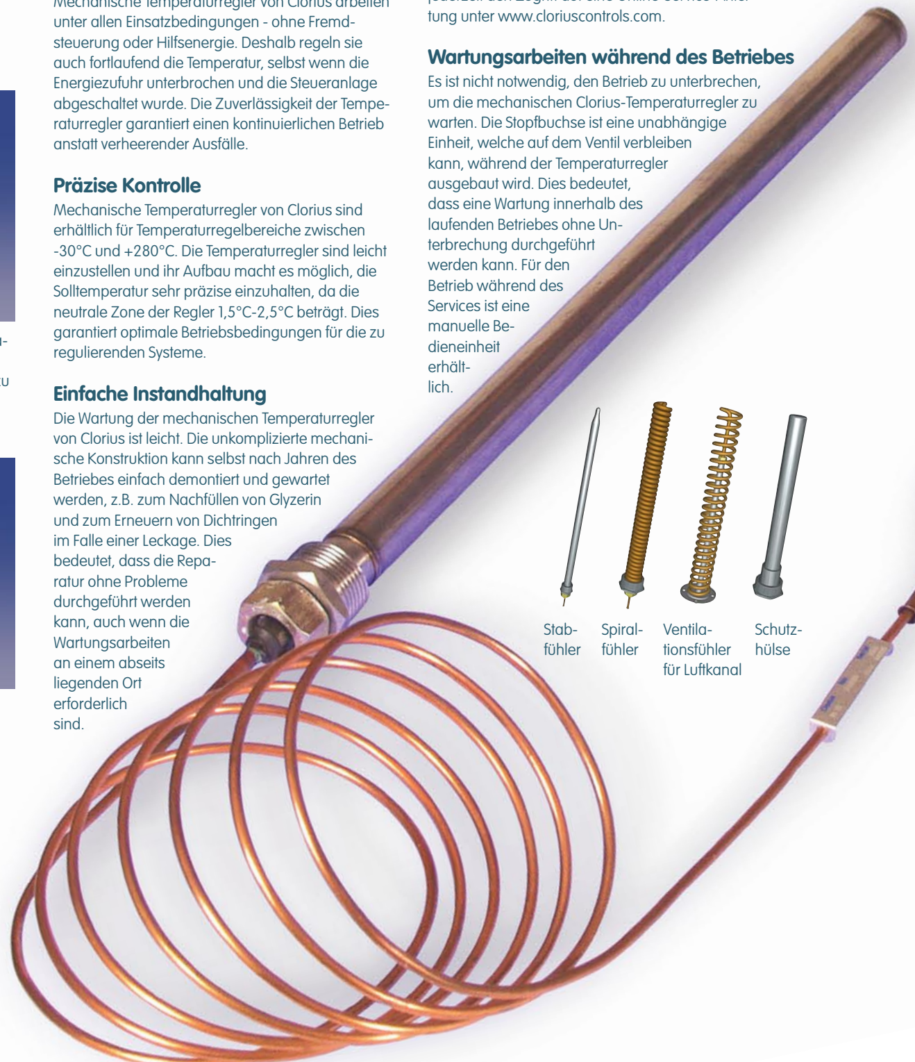
Die Sensorflüssigkeit (z.B. Glycerin) kann im Falle einer Leckage nachgefüllt werden.
